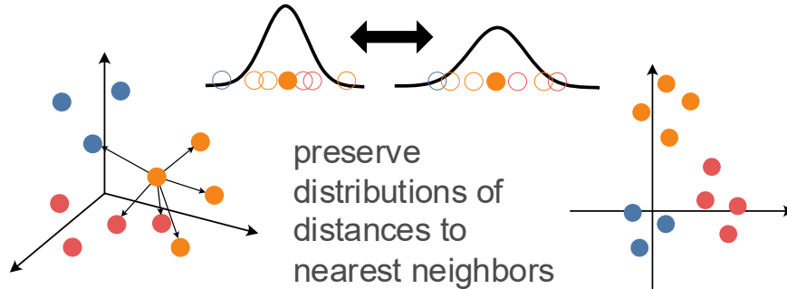
tSNE
