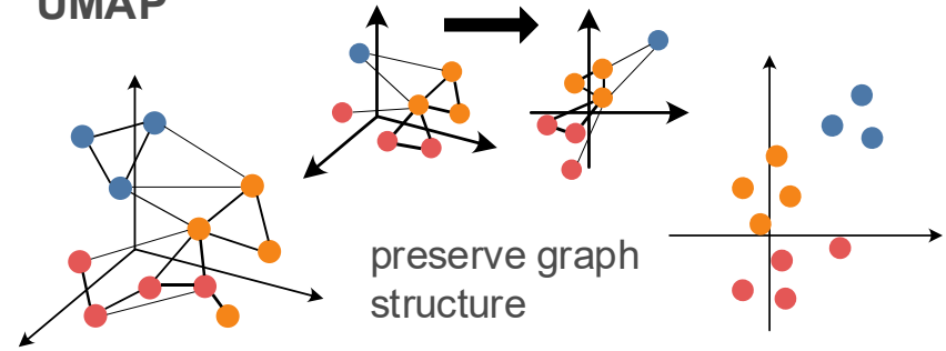
UMAP
